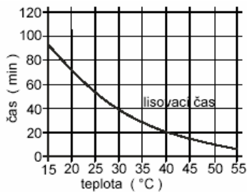
Diagram 2: lisovací čas
