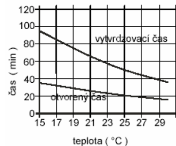
Diagram 1: Otvorený a vytvrdzovací čas pre SikaForce-7110 L55
