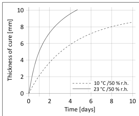
Graf: Rýchlosť vytvrdzovania SikaTack® Ultrafast
