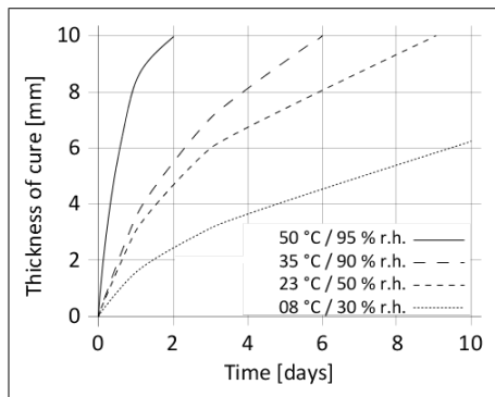
Graf 1: Rýchlosť vytvrdzovania Sikasil® AS-70
