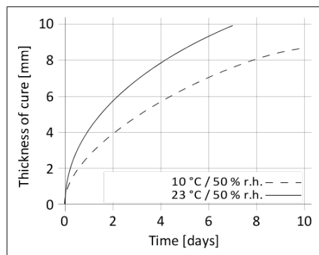
Graf 1: Rýchlosť vytvrdzovania SikaTack® PRO
